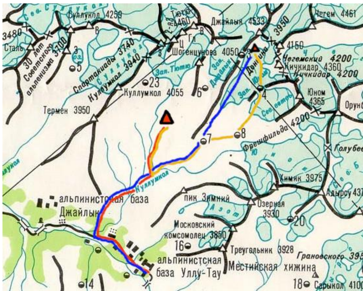
Рис. 1: Карта-схема района. На схеме отмечены ночевки, а также пути подхода и спуска.
