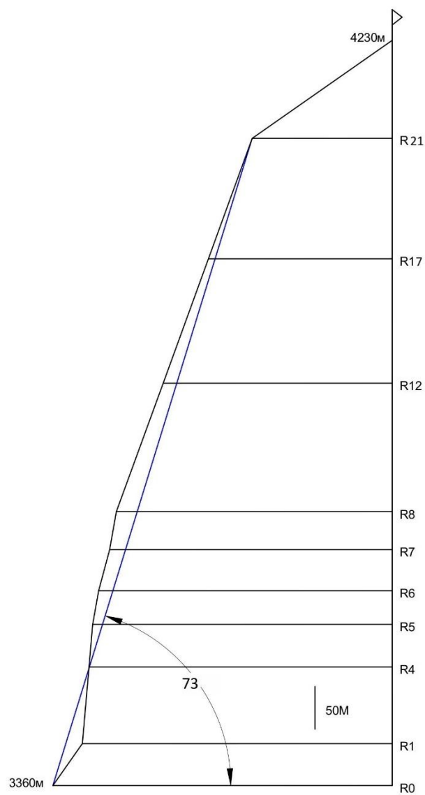
Профиль маршрута
