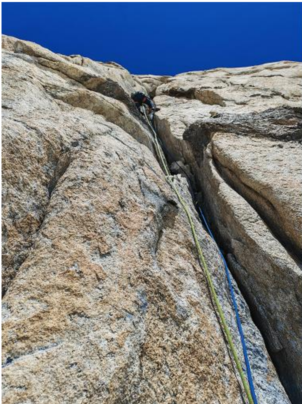
Рис. 3.9 – Участок R7 – R8. Ключевой участок скальной части маршрута
